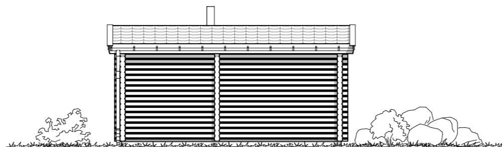
NORD FASADE
