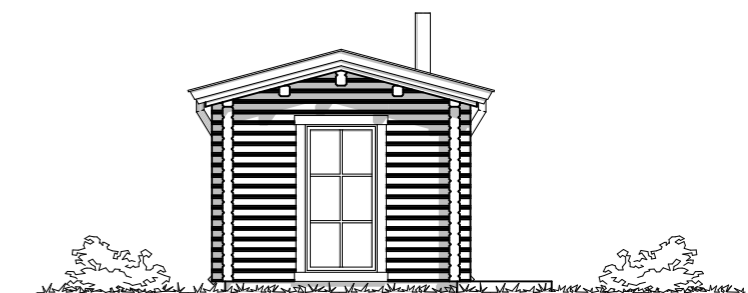
VEST FASADE
